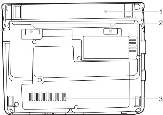
图 2-5. LifeBook U 系列笔记本底面板
