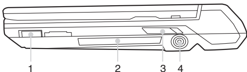
图 2-3. LifeBook U 系列笔记本右侧面板
